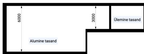
ÄRIPINNA SKEMAATILINE LÕIGE
